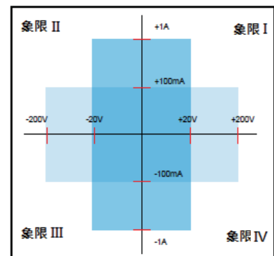
2450 功率包絡。
